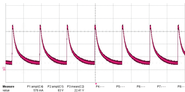
图28 – 输出电压: 230 VAC。 V_{OUT} , 20 V/格, 1 s/格
