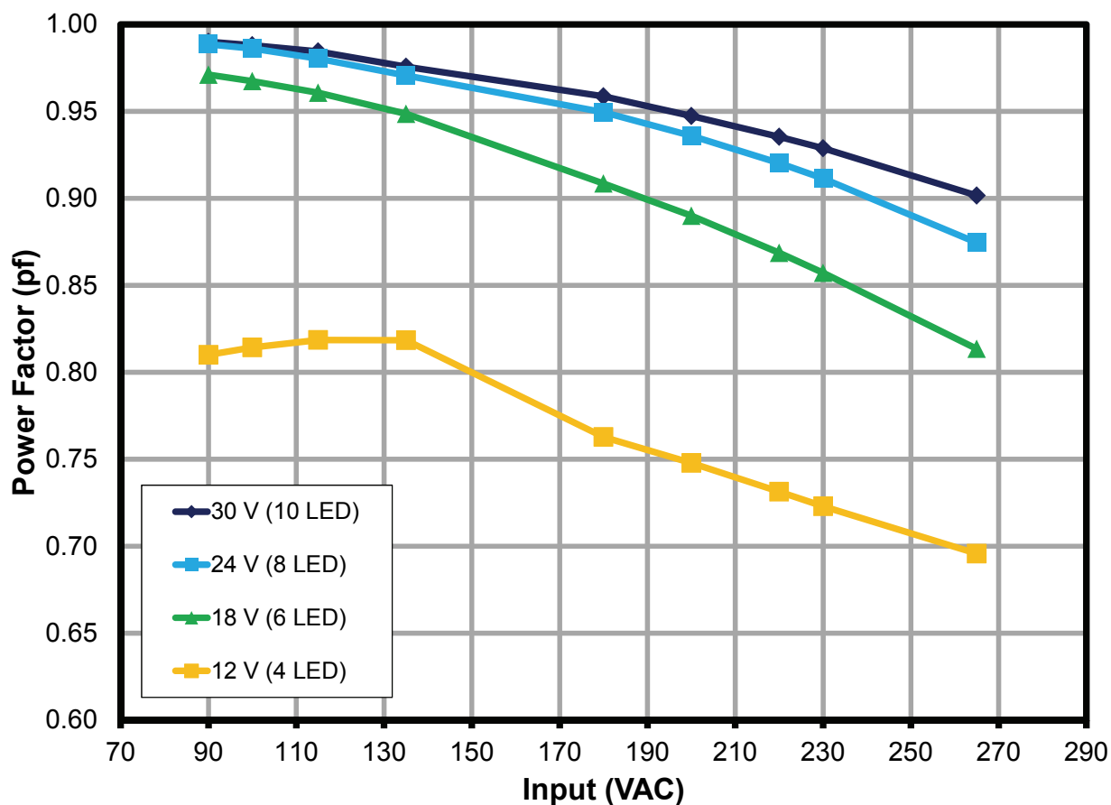
图11 – 功率因数随输入电压的变化，室温
