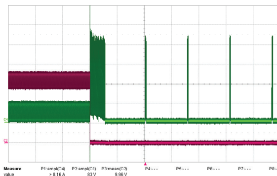
图26 – 110 VAC, 满载 上: I_{OUT} , 1 A/格 下: V_{DRAIN} , 10 V, 1 s/格
