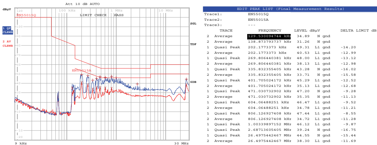
图30 – 传导EMI, 最大稳态负载, 110 VAC, 相线, 60 Hz, EN55015 B限值
