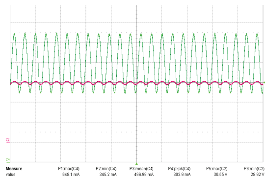
图20 – 115 VAC, 满载 上: I_{OUT} , 100 mA/格 下: V_{OUT} , 10 V, 5 ms/格
