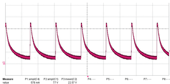
图27 – 输出电压: 110 VAC。 V_{OUT} , 20 V/格, 1 s/格
