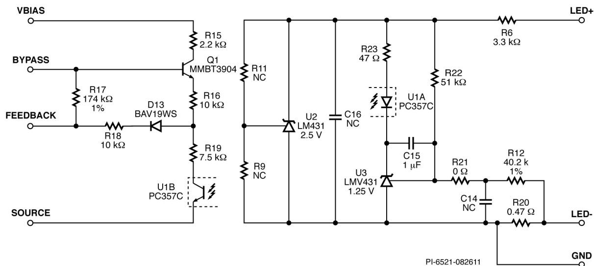
图33 – 图6中所示的PCB布局电路图
