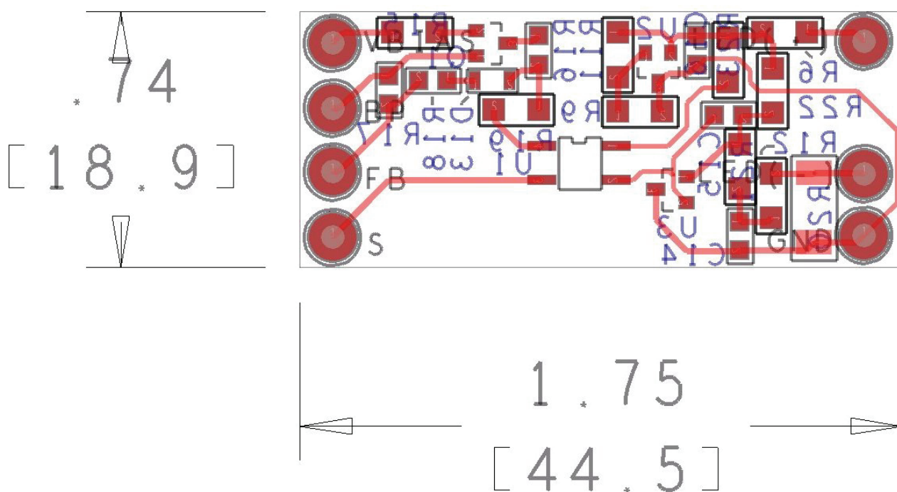
图6 – 次级恒流调节子板的PCB布局（与该布局相匹配的实际电路原理图见附录A）
