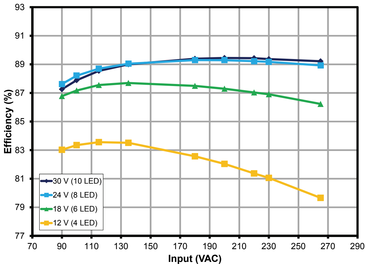
图9 – 不同LED负载在不同输入电压下的效率图
