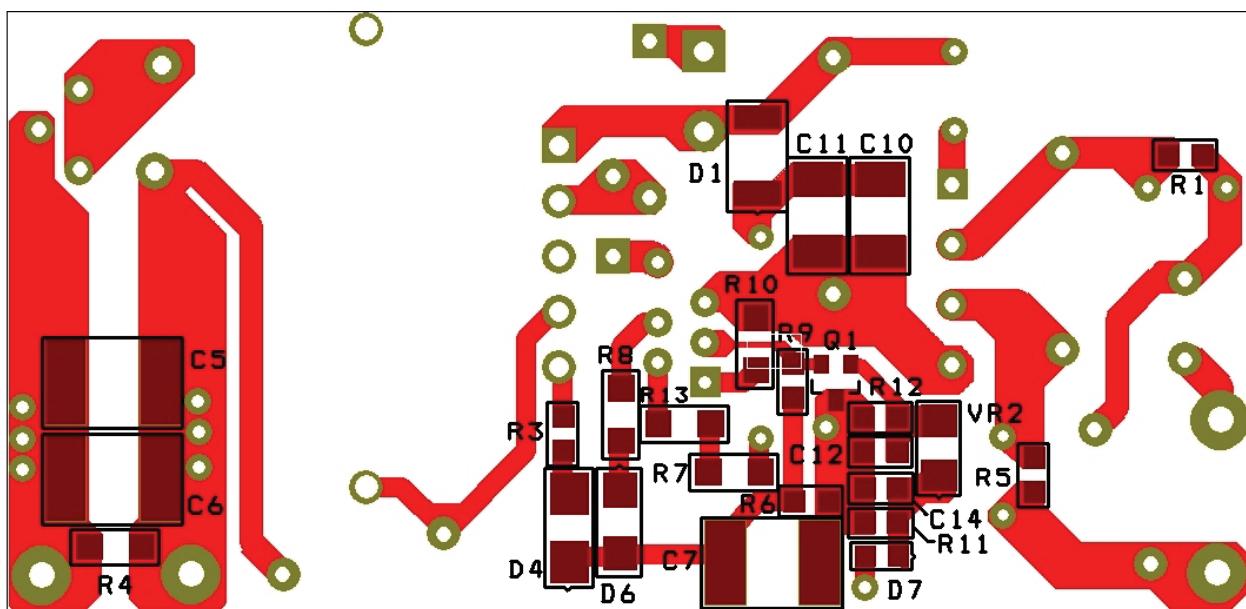
图5 – DER-289板PCB布局，底视图
