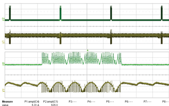
图25 – 265 VAC, 满载 上: I_{OUTPUT} , 2 A/格 下: V_{DRAIN} , 200 V, 500 ms/格
