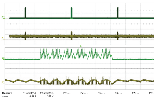
图24 – 90 VAC, 满载 上: I_{OUTPUT} , 2 A/格 下: V_{DRAIN} , 200 V, 500 ms/格
