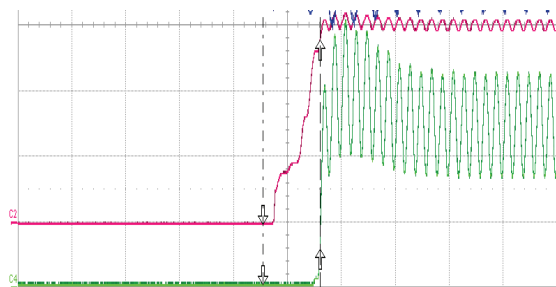
图18 – 115 VAC, 满载 上: V_{OUT} , 10 V, 5 ms/格 下: I_{OUT} , 100 mA/格
