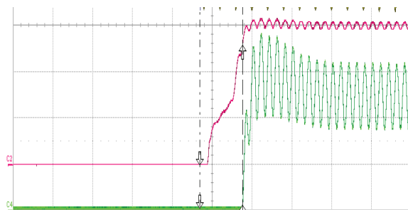
图19 – 230 VAC, 满载 上: V_{OUT} , 10 V, 5 ms/格 下: I_{OUT} , 100 mA/格
