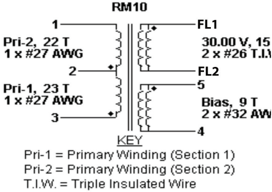
图7 – 变压器电气原理图。
