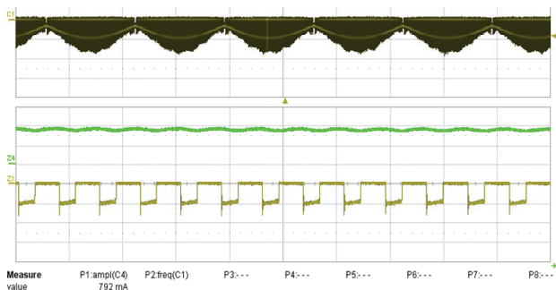
图22 – 110 VAC, 满载 上: I_{RIPPLE} , 0.5 A/格 下: V_{DIODE} , 100 V, 5 ms/200 \mu s/格
