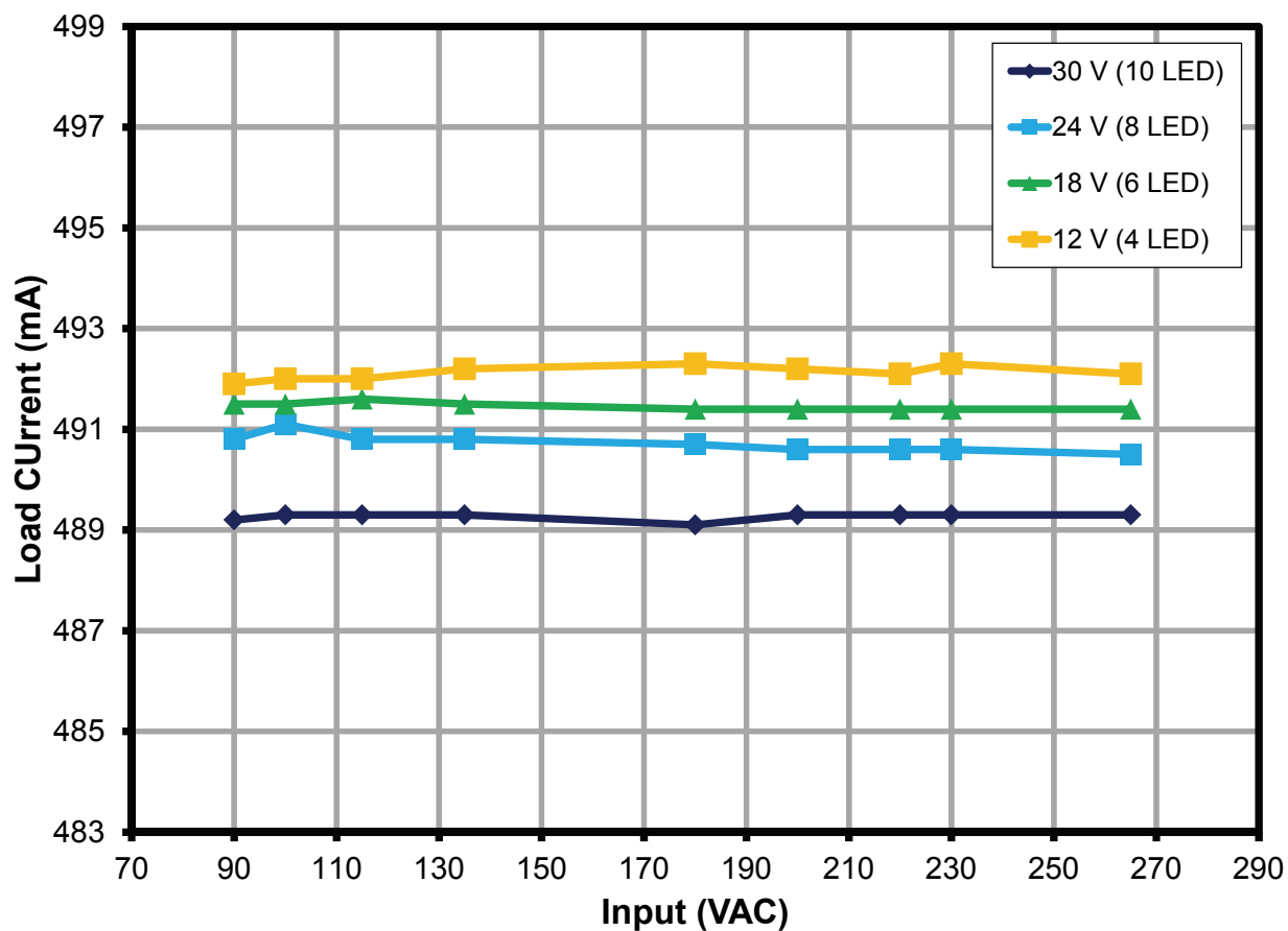
图10 – 不同LED负载在不同输入电压下的电压调整率，室温
