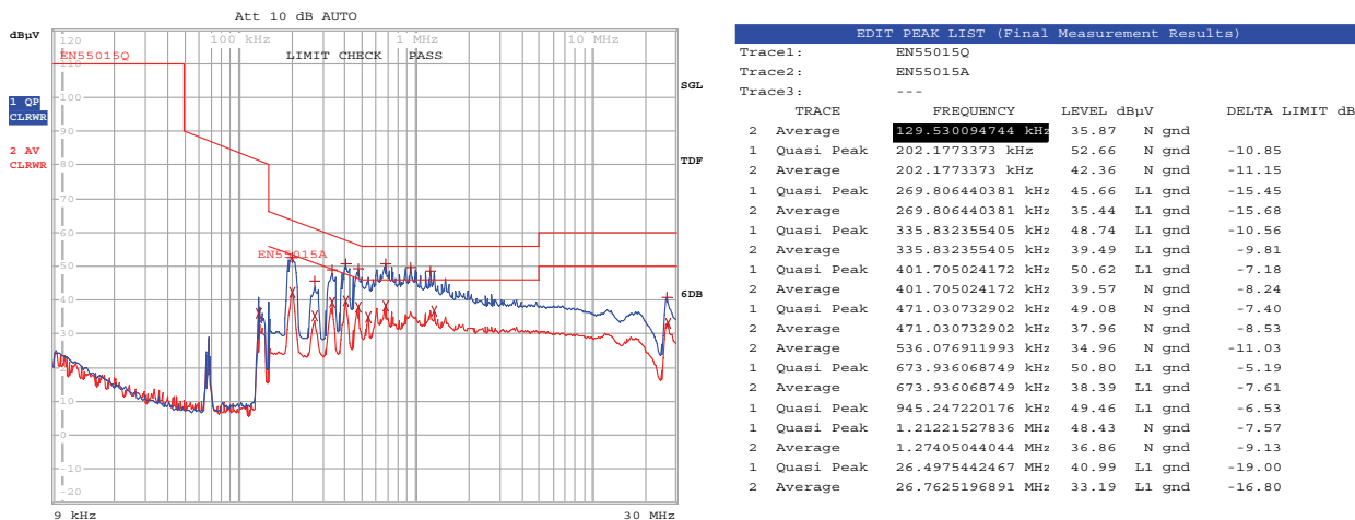
图32 – 传导EMI，最大稳态负载，230 VAC，零线，60 Hz，EN55015 B限值
