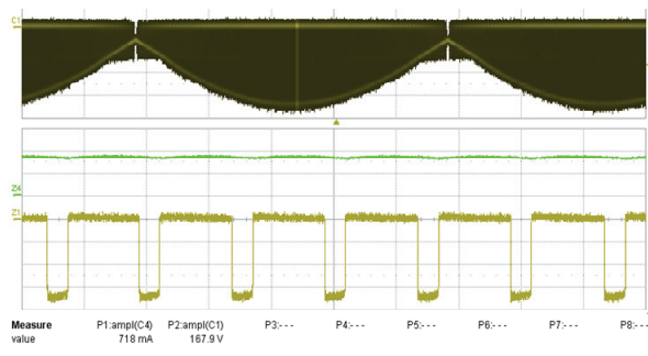
图23 – 265 VAC, 满载 上: I_{RIPPLE} , 0.5 A/格 下: V_{DIODE} , 100 V, 5 ms/200 \mu s/格
