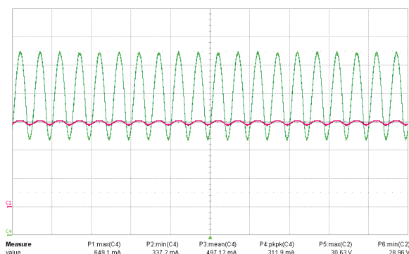
图21 – 230 VAC, 满载 上: I_{OUT} , 100 mA/格 下: V_{OUT} , 10 V, 5 ms/格
