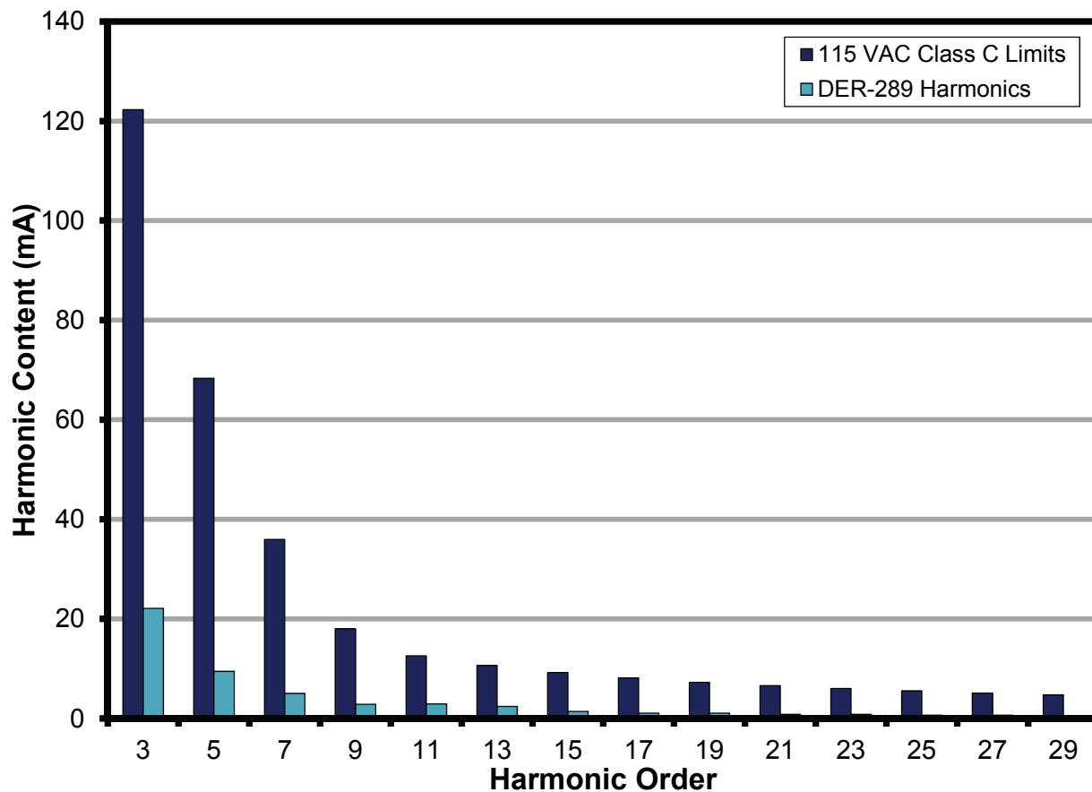
图12 – 115 VAC谐波，室温，满载
