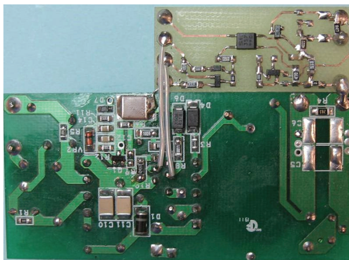
图1 – 参考板DER-284和 次级恒流调节子板（顶视图）
