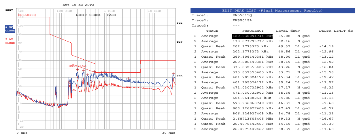
图31 – 传导EMI，最大稳态负载，110 VAC，零线，60 Hz，EN55015 B限值
