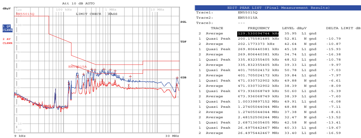
图29 – 传导EMI, 最大稳态负载, 230 VAC, 相线, 60 Hz, EN55015 B限值
